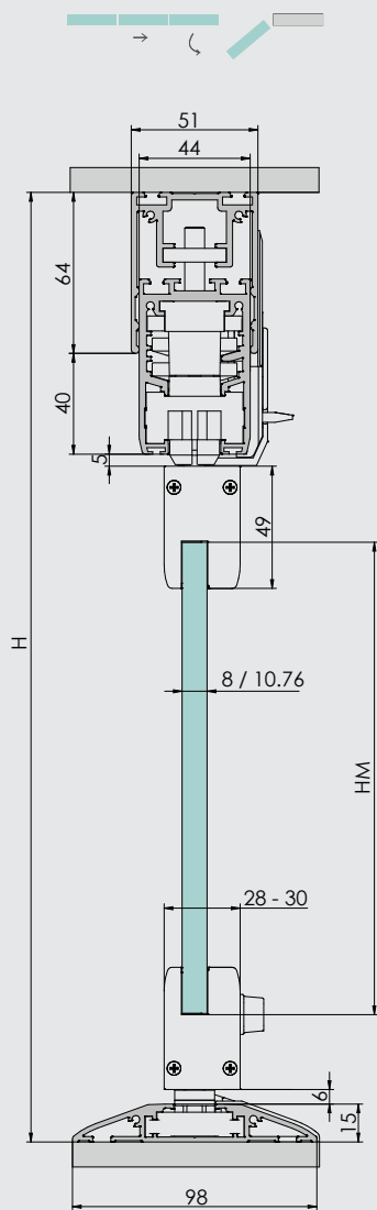
Znižano spodnje vodilo H15 mm
