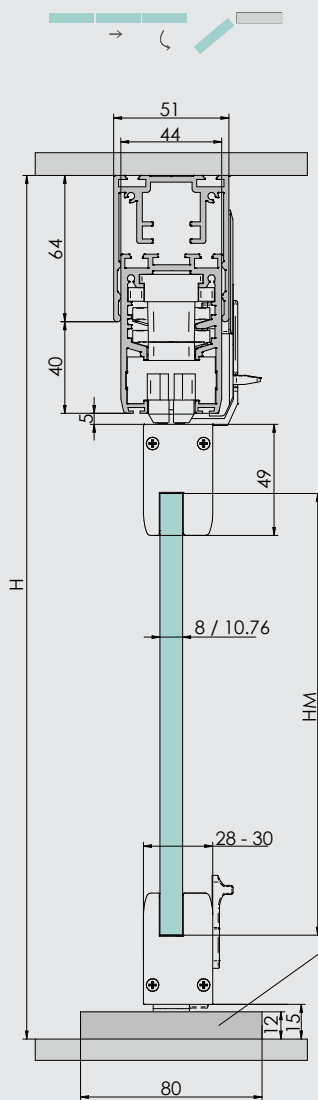
Brez spodnjega vodilo H00 mm
